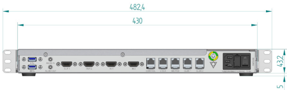
ラック寸法（オプション） Rack Dimensions (optional)
